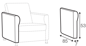
armrest 8200
