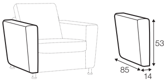
armrest 7000
